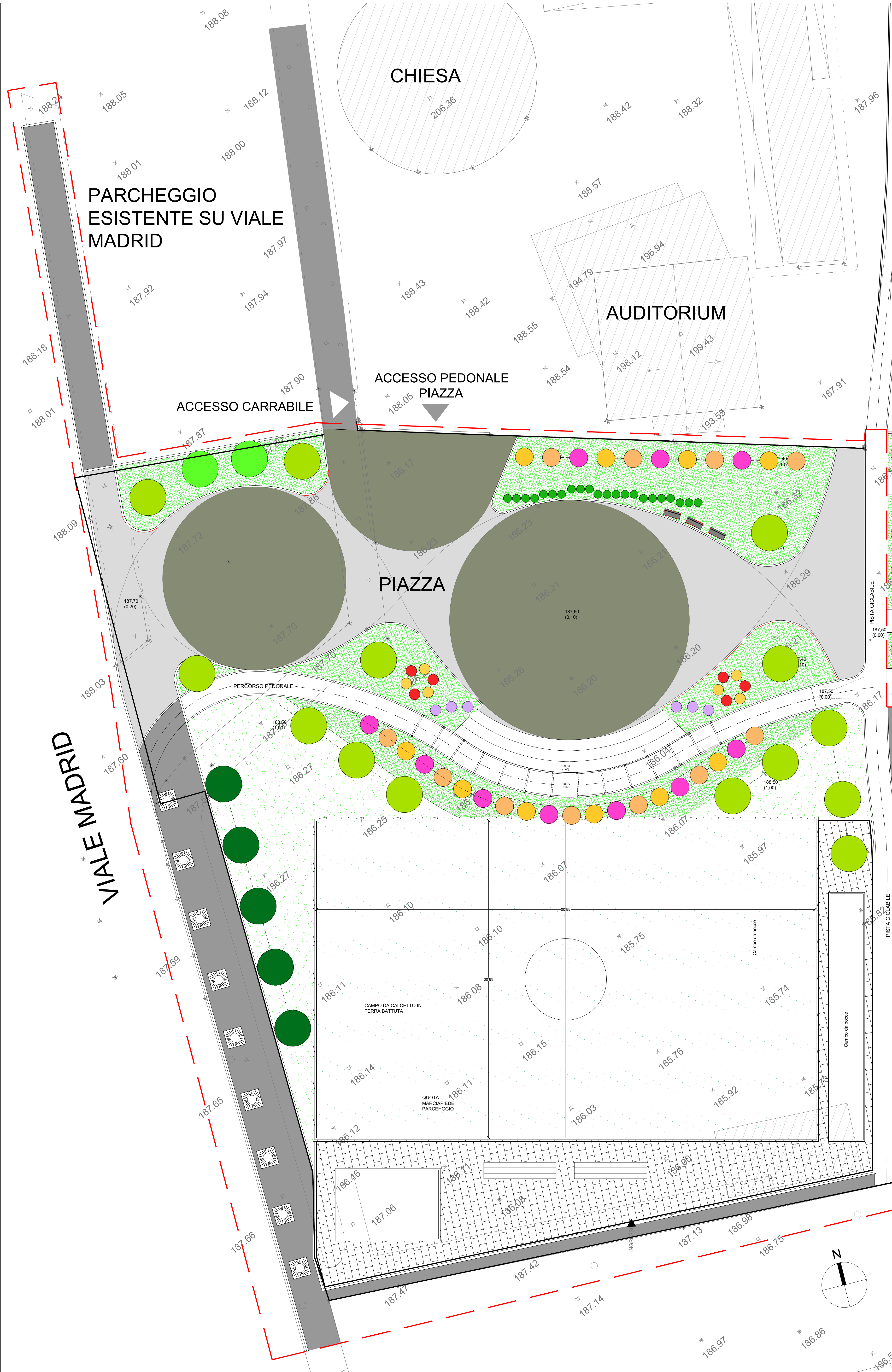
AREA VERDE ATTREZZATO 8 POST OPERAM - scala 1:200
